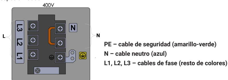
Figura 20. Conexión del equipo a la instalación eléctrica
