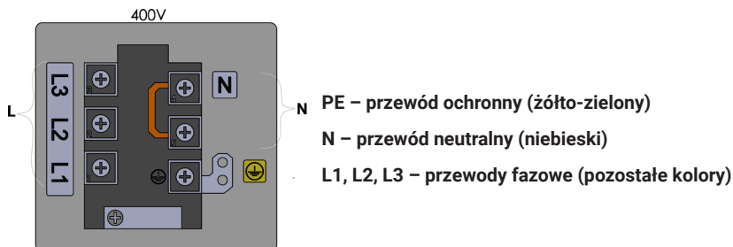
Rysunek 20. Podłączenie urządzenia do instalacji elektrycznej
