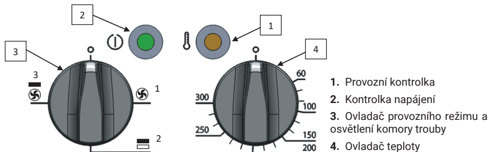
Obrázek 14. Eco ovládání trouby
