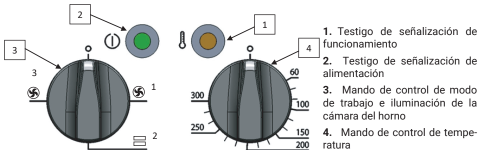
Figura 13. Controles del horno ECO
