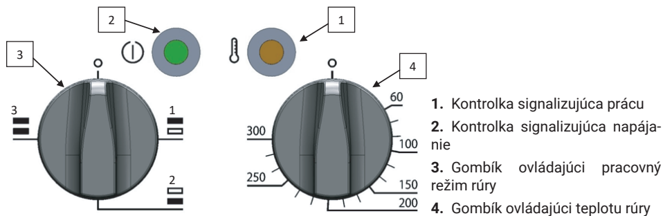
Obrázok 12. Ovládacie prvky statickej rúry
