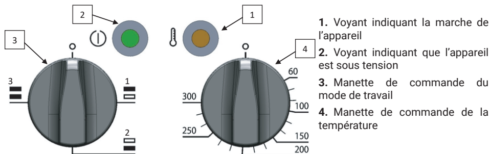
Figure 12. Composants du système de commande du four statique
