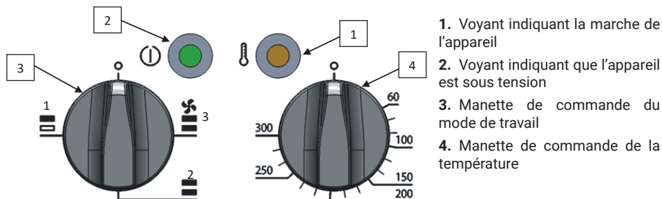
Figure 11. Composants du système de commande du four – 3 systèmes de chauffe
