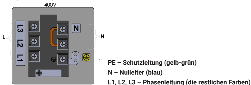
Bild 20. Anschluss des Gerätes an die elektrische Installation
