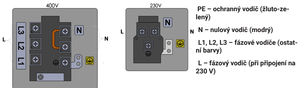
Obrázek 21. U sporáku ECO musí být spotřebič připojen do elektrické sítě podle štítku na spotřebiči.
