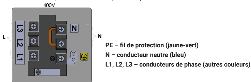
Figure 20. Connexion de l'appareil au réseau électrique
