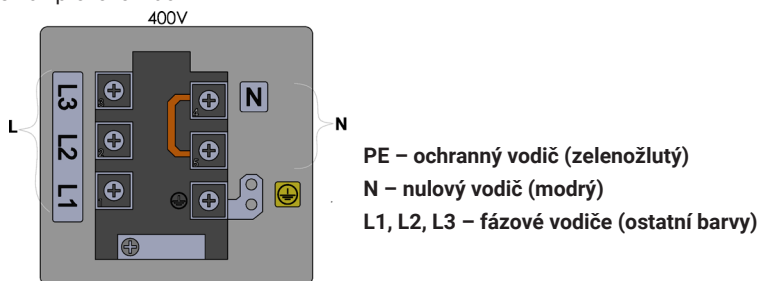
Obrázek č. 20. Připojení zařízení k elektrické síti
