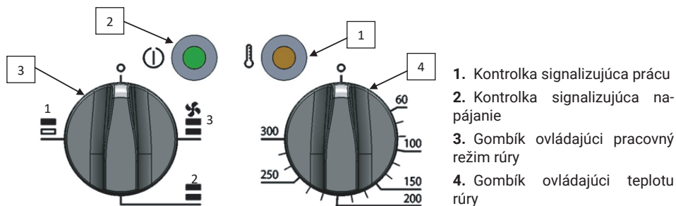
Obrázok 11. Ovládacie prvky rúry - 3 systémy ohrievania
