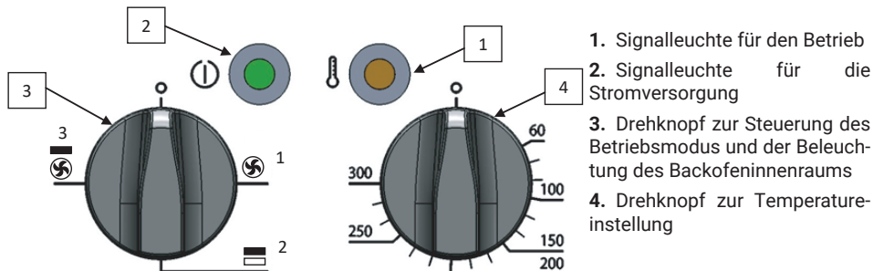
Bild 14. ECO-Ofen-Steuerungen
