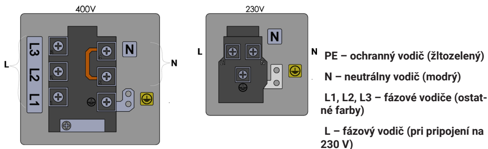
Obrázok 21. Pripojenie spotrebiča k elektrickej inštalácii pre sporák ECO podľa štítiku na zariadení.
