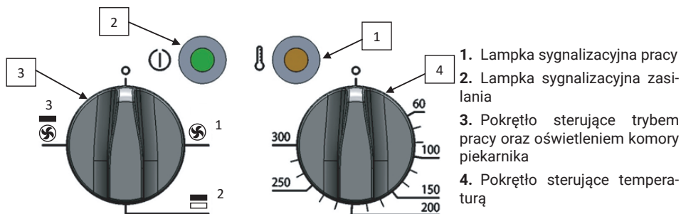
Rysunek 14. Elementy sterujące piekarnika ECO
