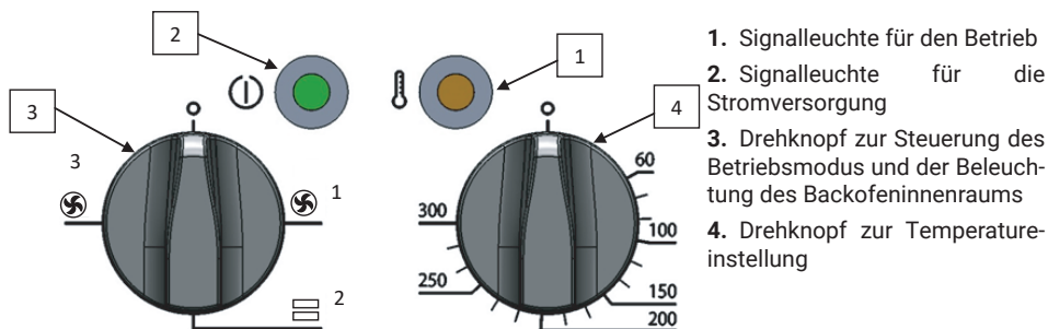
Bild 13. ECO-Ofen-Steuerungen
