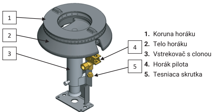
Obrázok 18. Konštrukcia horáku na príklade horáku 7kW.
