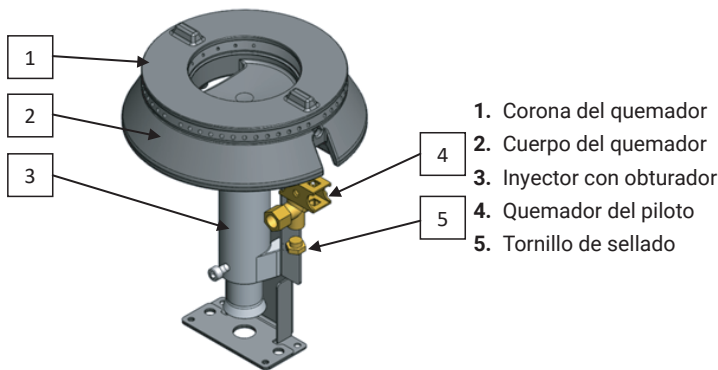
Figura 18. Diseño del quemador sobre el ejemplo de un quemador de 7 kW
