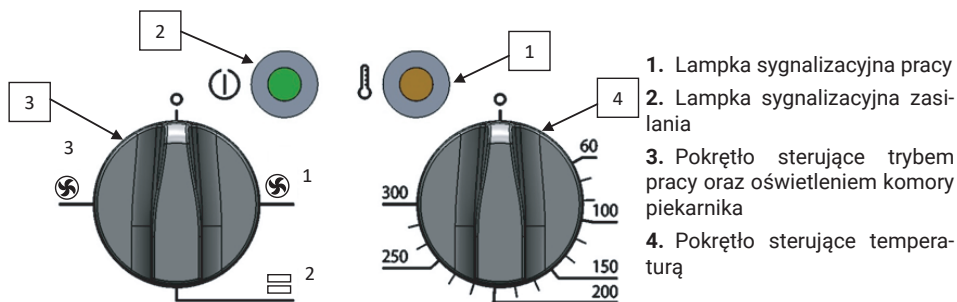
Rysunek 13. Elementy sterujące piekarnika ECO
