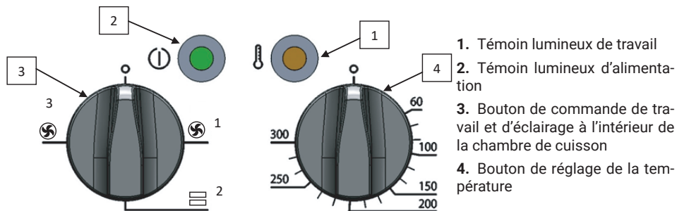
Figure 13. Contrôles des fours ECO
