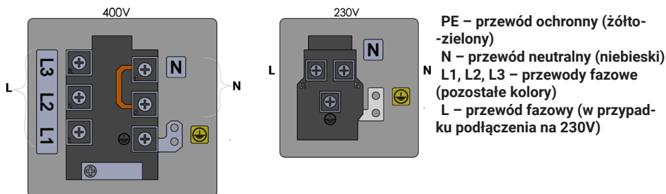
Rysunek 21. Podłączenie urządzenia do instalacji elektrycznej dla kuchni ECO zgodnie z etykietą na urządzeniu.
