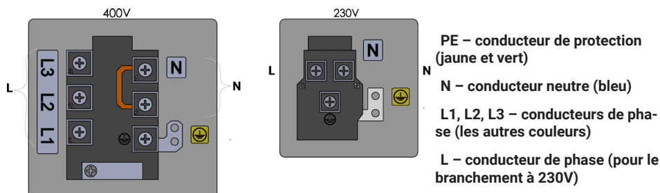
Figure 21. Branchement de l'appareil au réseau électrique pour la cuisinière ECO, conformément à l'étiquette sur l'appareil.
