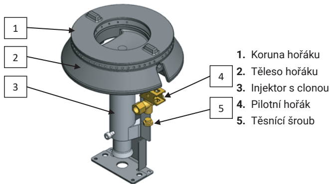
Obrázek č 18. Konstrukce hořáku na příkladu 7kW hořáku.
