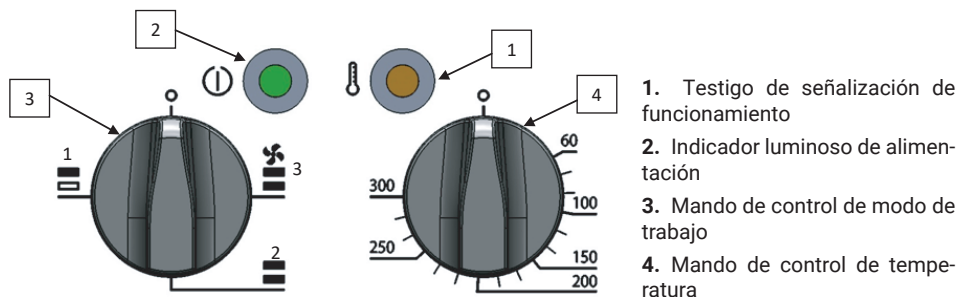
Figura 11. Elementos de control del horno – 3 sistemas de calentamiento
