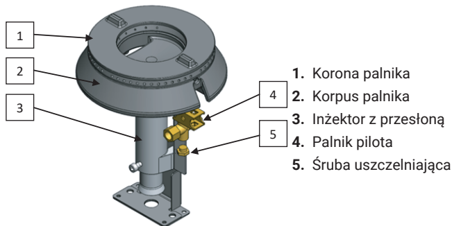
Rysunek 18. Budowa palnika na przykładzie palnika 7kW.
