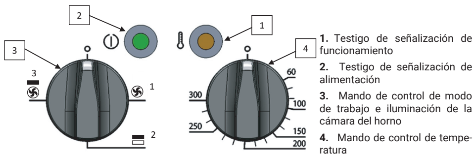
Figura 14. Controles del horno ECO
