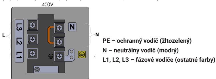
Obrázok 20. Pripojenie zariadenia k elektrickej sieti
