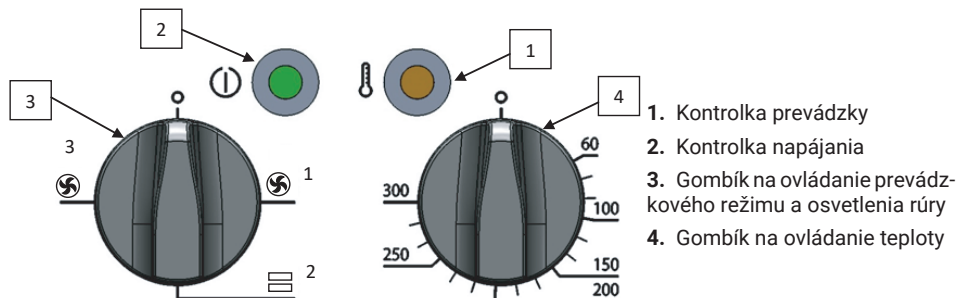
Obrázok 13. Ovládacie prvky pece ECO
