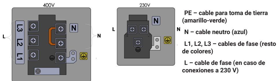
Figura 21. Conexión del equipo a la instalación eléctrica para cocina ECO según la etiqueta del dispositivo.
