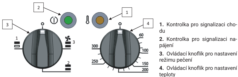
Obrázek č 11. Ovládací prvky pečící trouby – 3 režimy pečení
